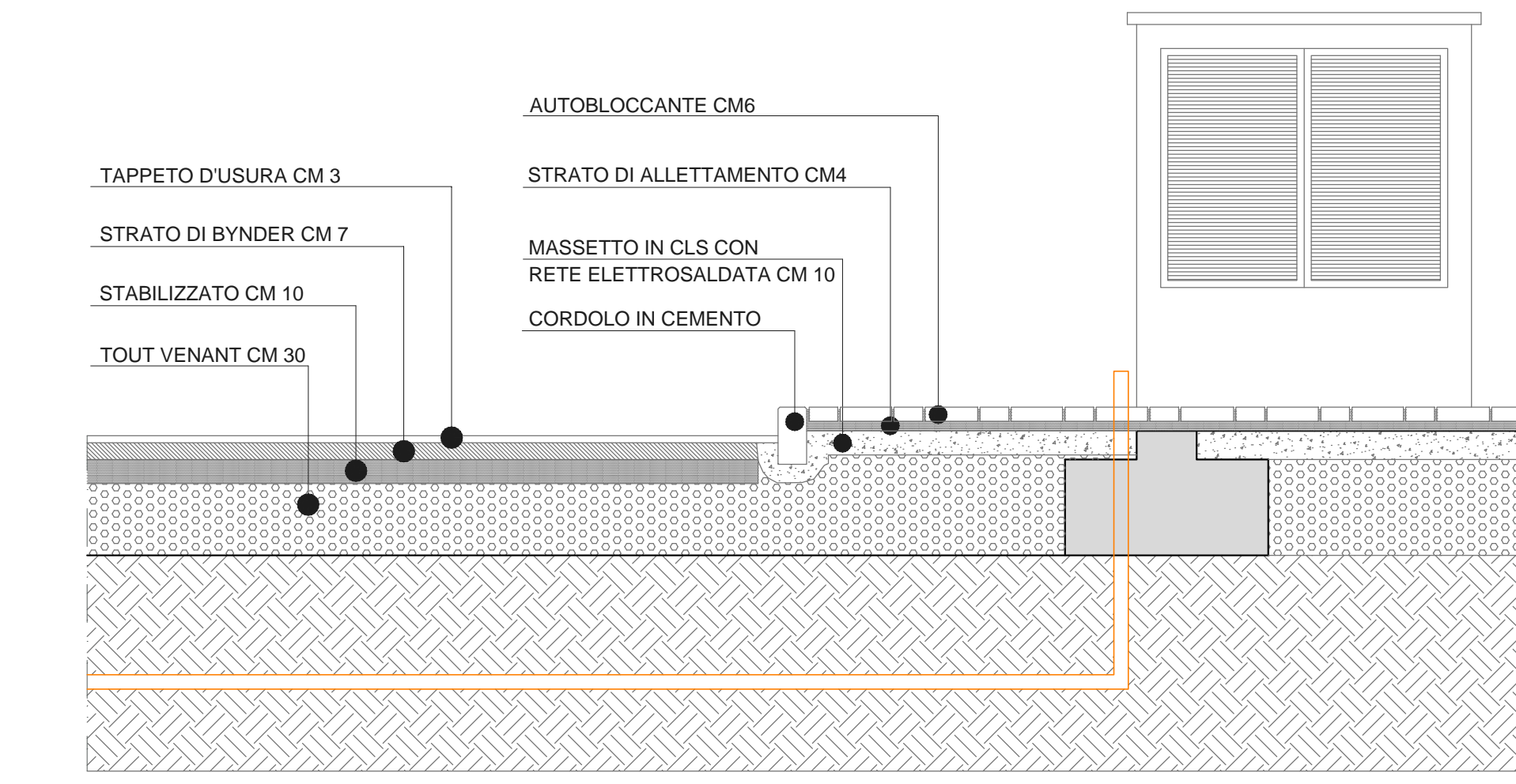
VISTA NICCHIA TIPO GAS METANO Sc. 1:20
