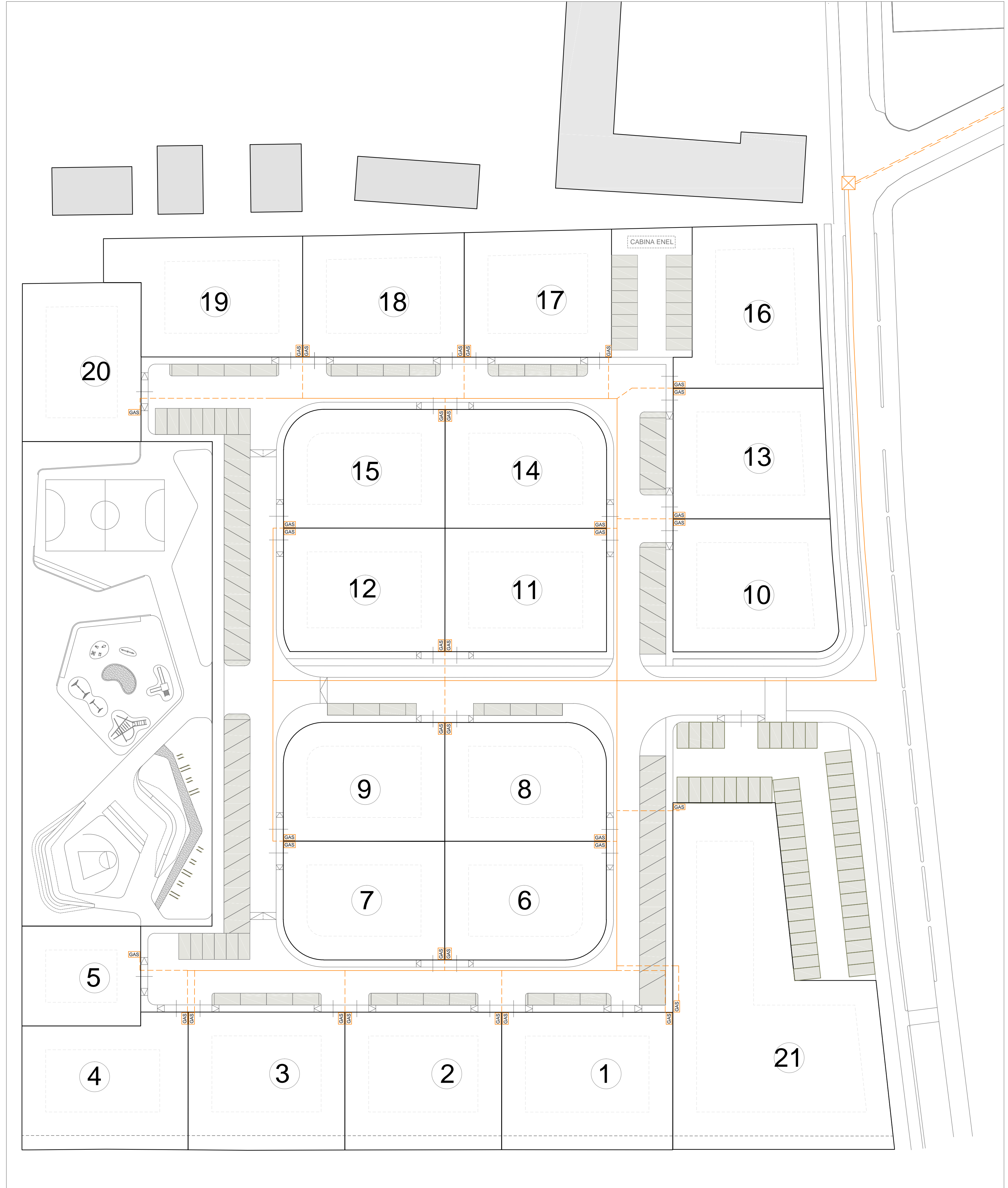
PLANIMETRIA GENERALE LOTTIZZAZIONE - Sc. 1:500
